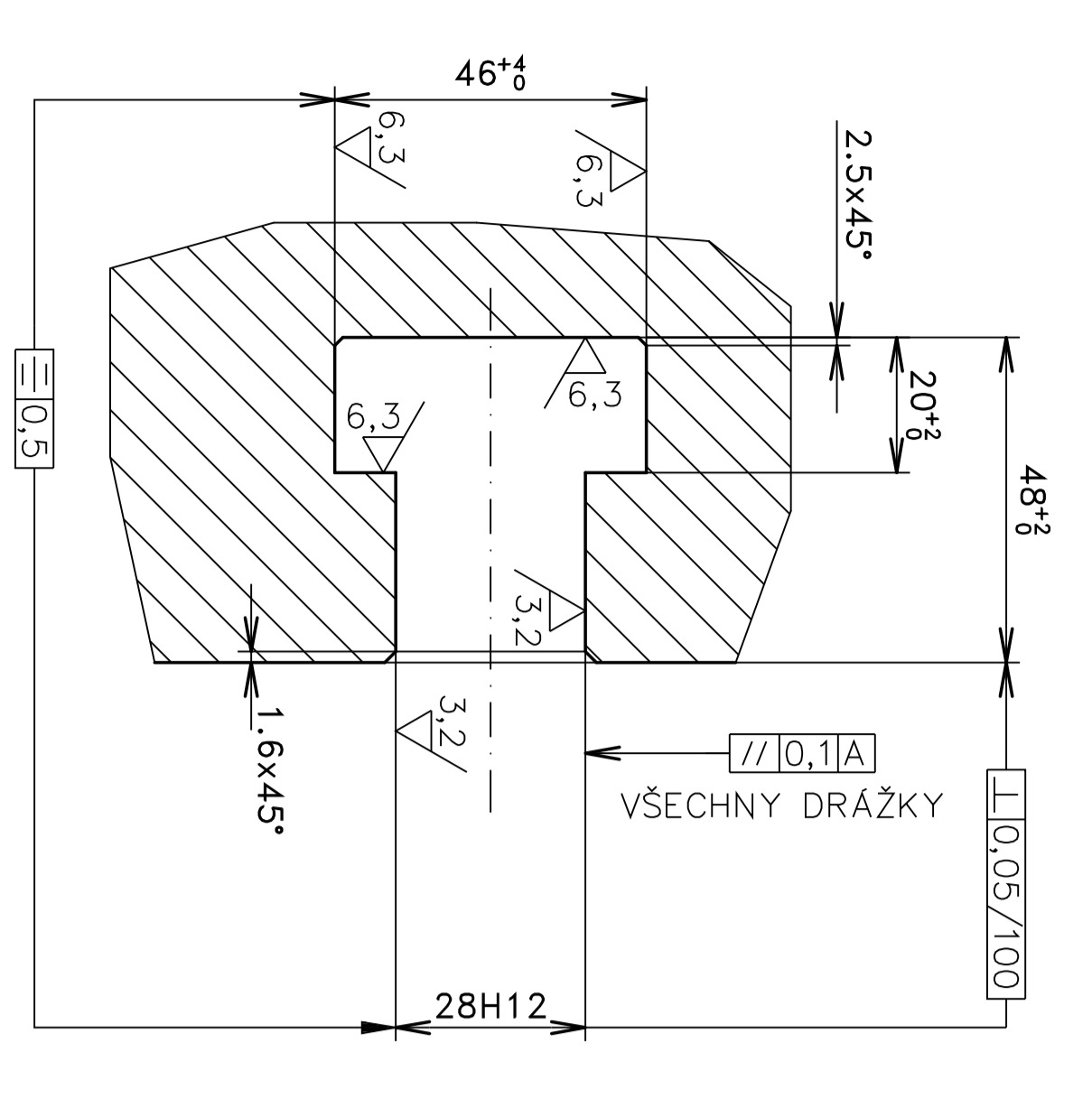
DETAIL D M 1:1
